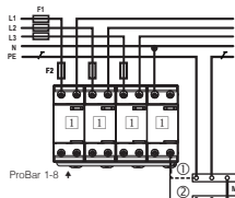
TN-S system, V-connection (only if F1 ≤ 100A)
