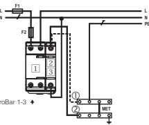
TT system, V-connection (only if F1 ≤ 100A)
