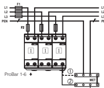
TN-C system, V-connection (only if F1 ≤ 100A)
