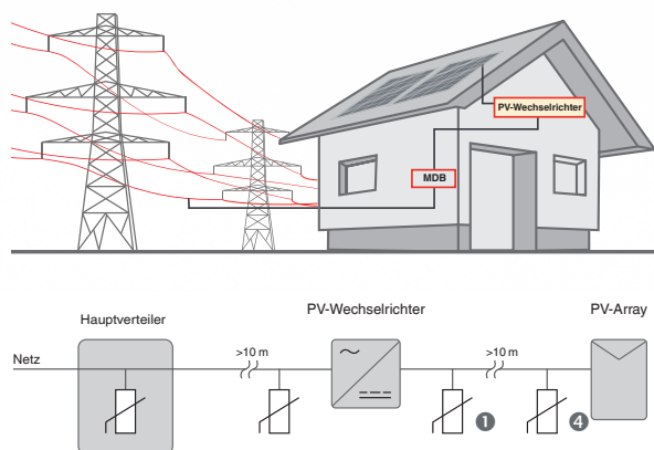
Abbildung 1: SPD 4 wird nicht benötigt, wenn die Kabellänge zwischen 1 und 4 < 10m ist
